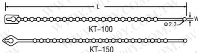
珠形束線帶KT系列產品工程圖
