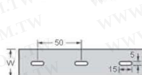
一般底槽固定孔 (W: 60mm 以下)
