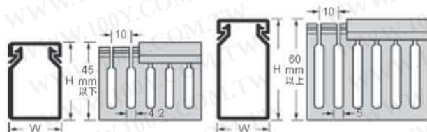
出線孔 S 型 (4.2mm 及 5mm)
