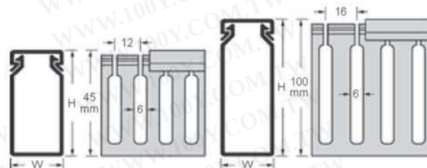
出線孔 M 型 (6mm)
