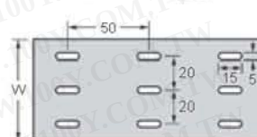
大型底槽固定孔 (W: 65mm 以上)
