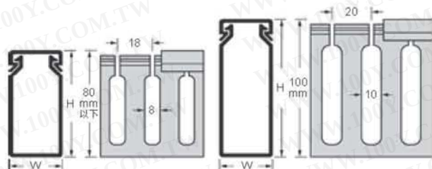
出線孔 L 型 (8mm 及 10mm)
