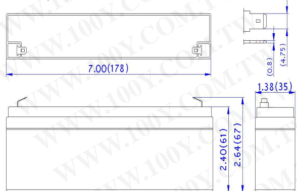
Unit:inch(mm)
