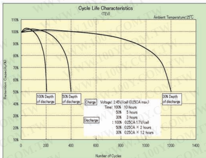
2. 循環使用壽命之特性 (Life Characteristics of Cycle Use)
