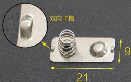
7号双极片 (21X9MM) 双向
